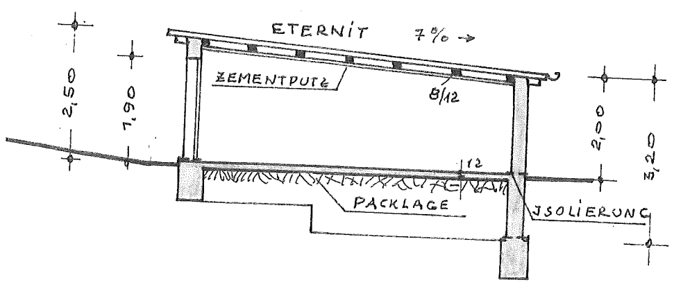
— SCHNITT DURCH GARAGE —
