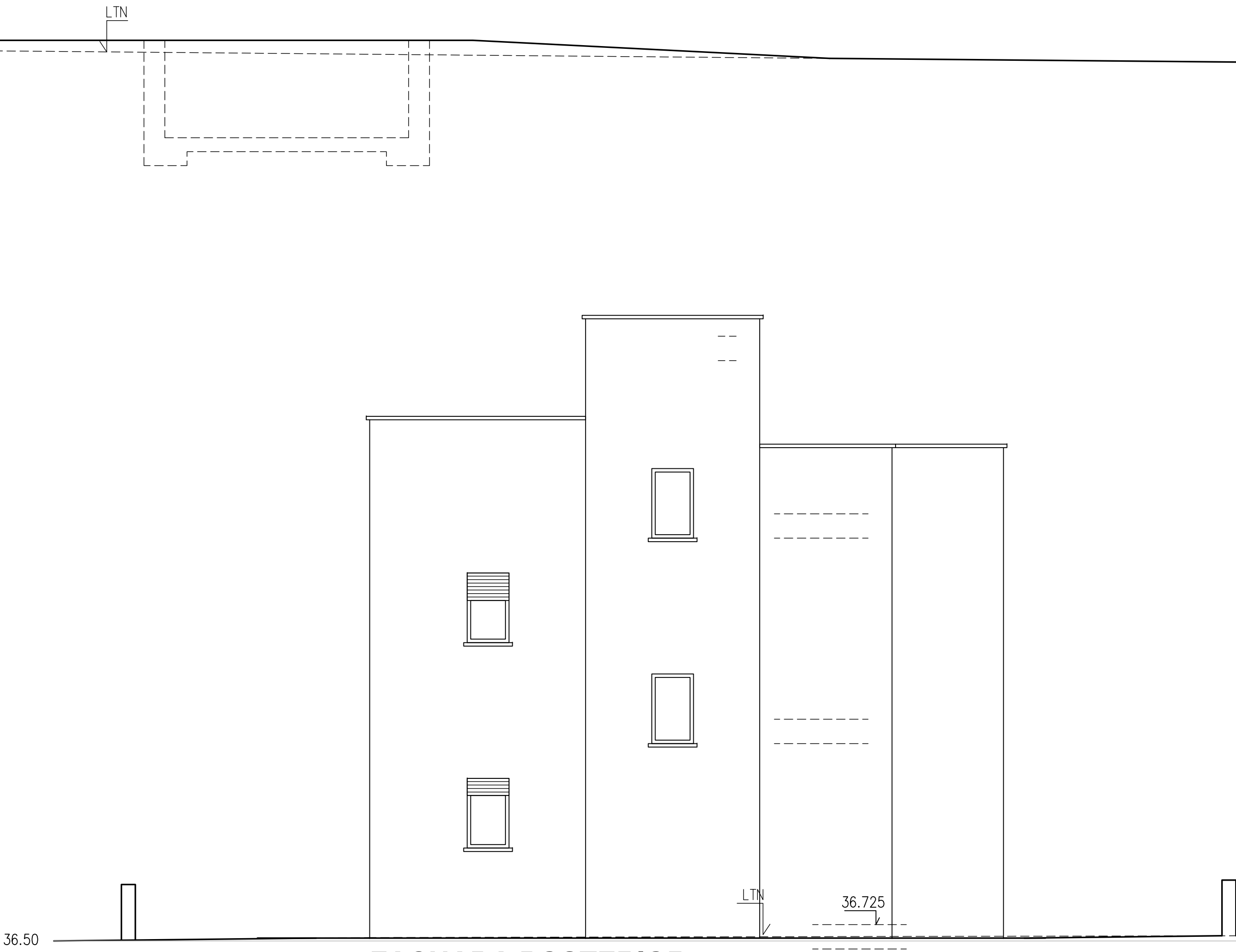
FACHADA POSTERIOR
