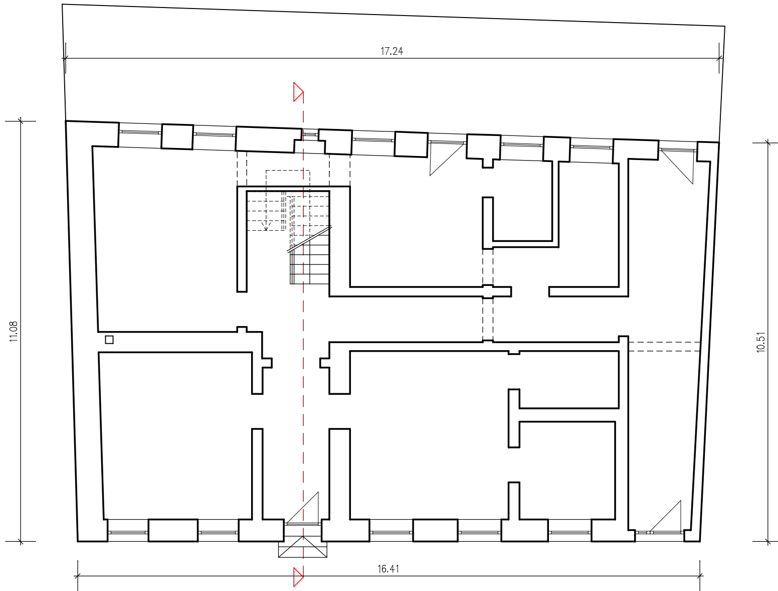
Erdgeschoss
