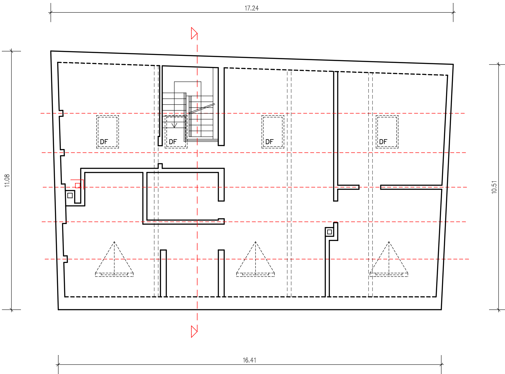
Dachgeschoss
