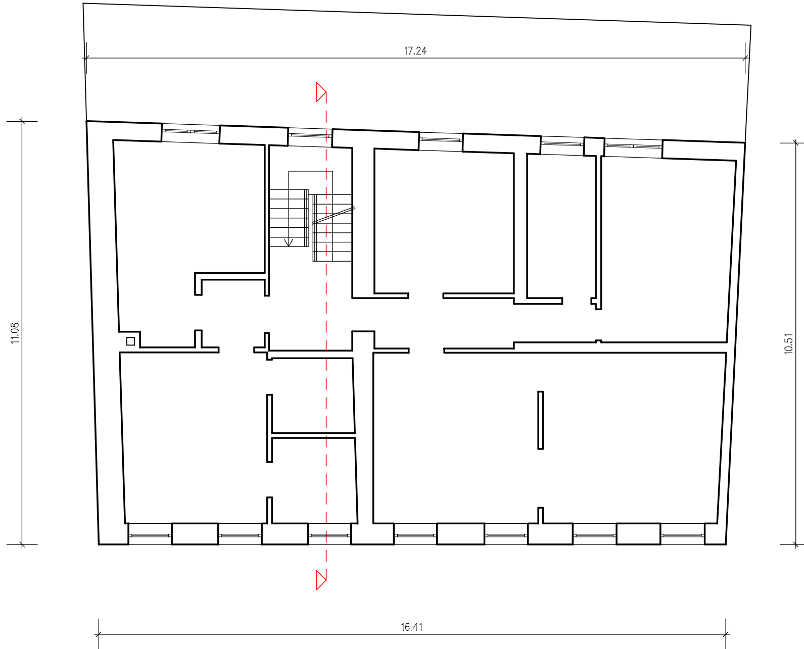
Obergeschoss
