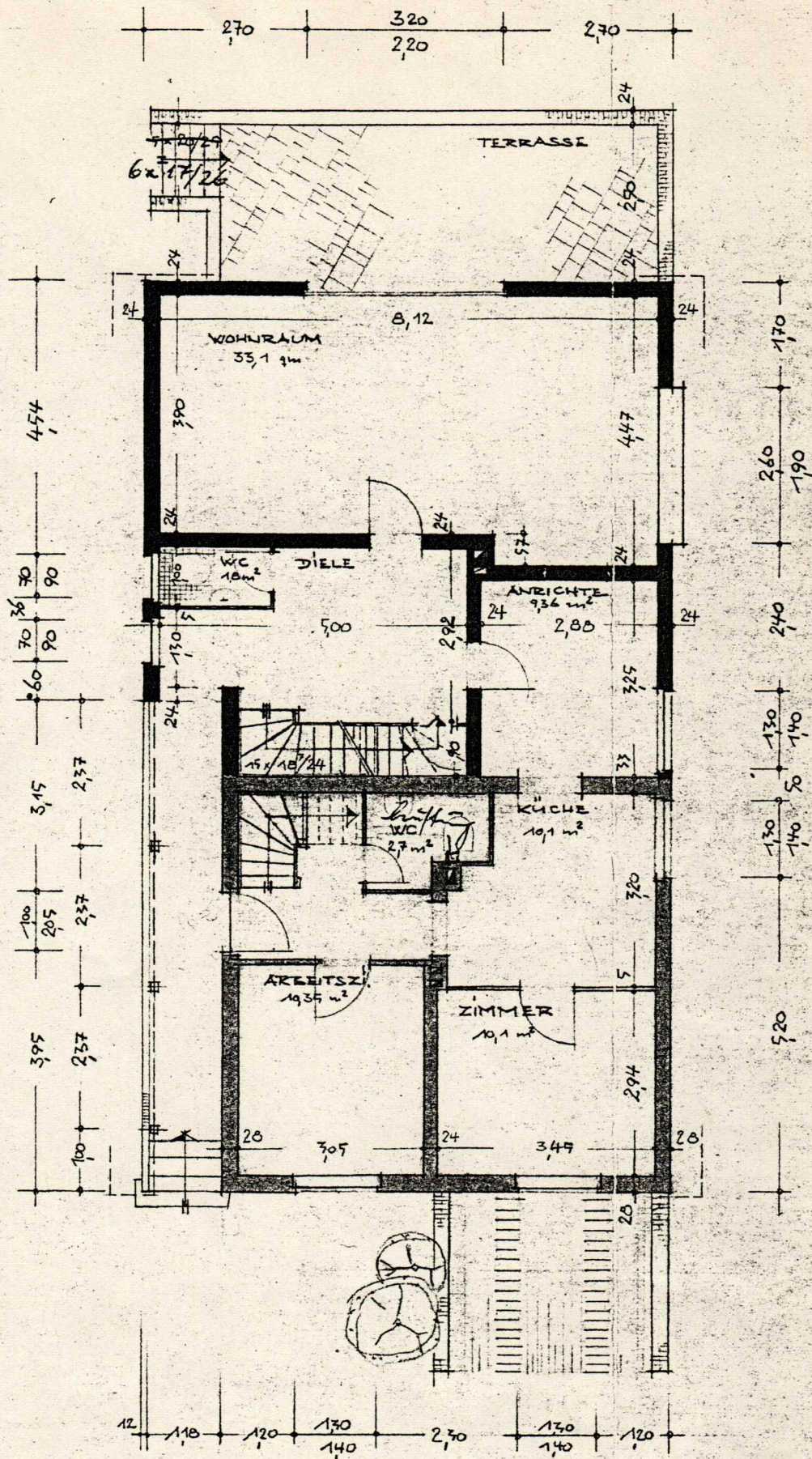
ERDGESCHOSS
