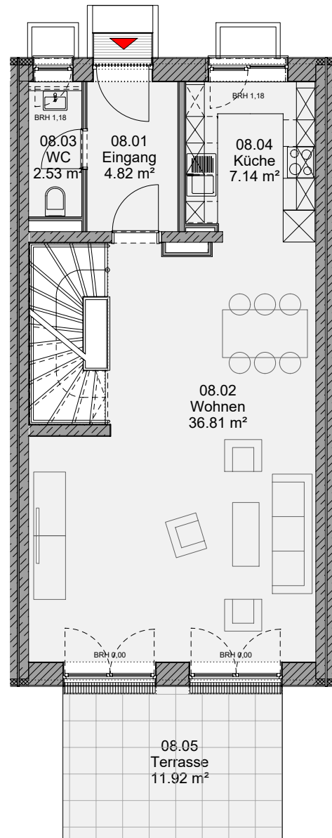
ERDGESCHOSS
