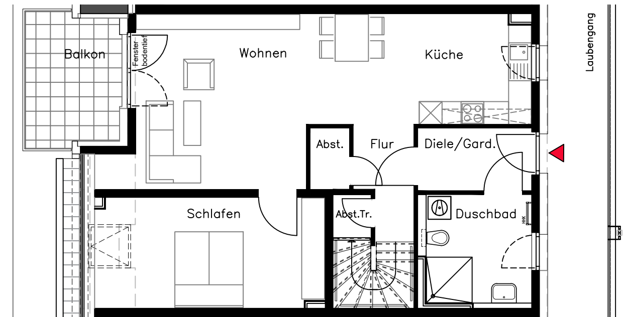
Wohnung A 9, DG
