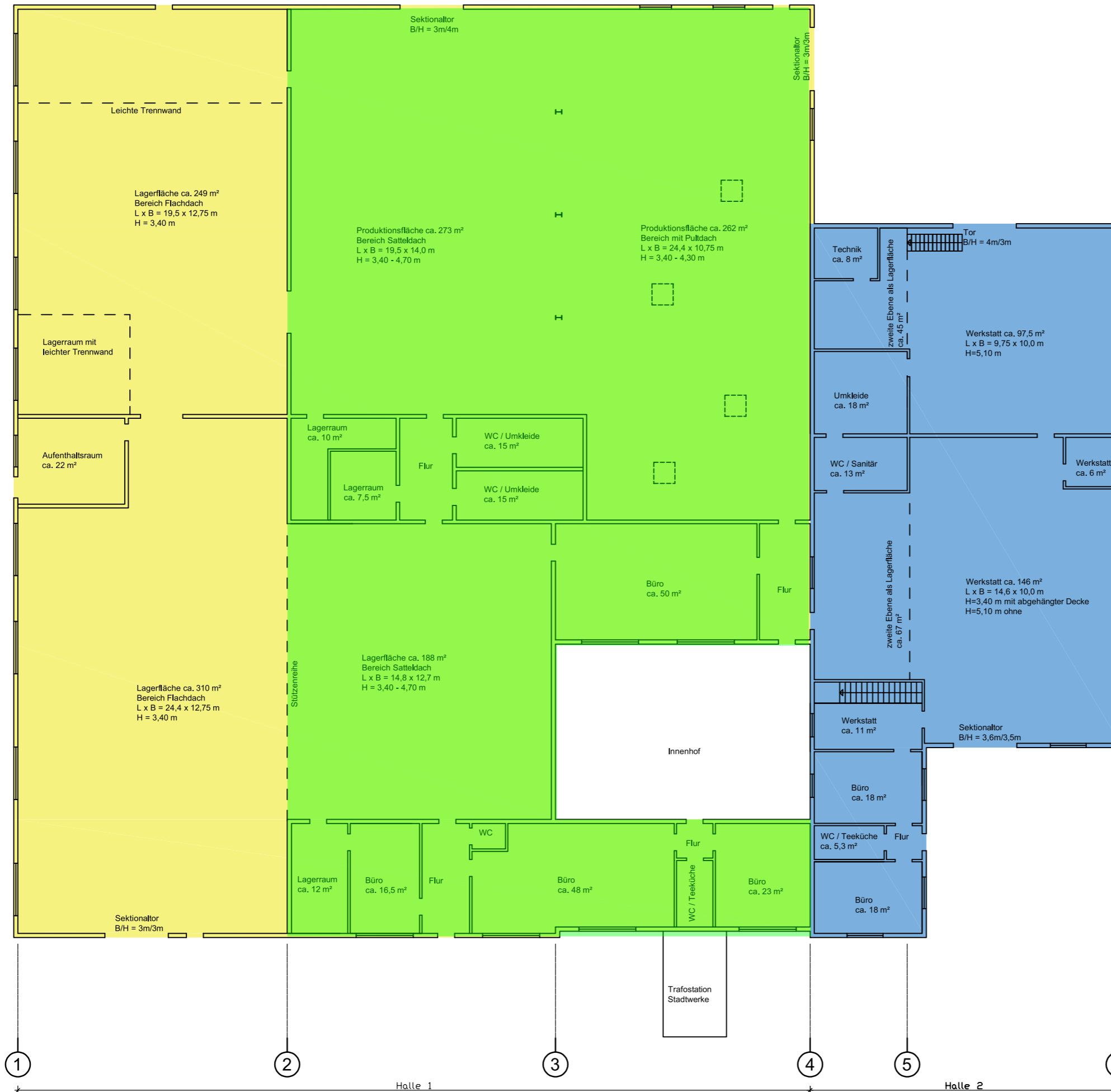
Grundriss
