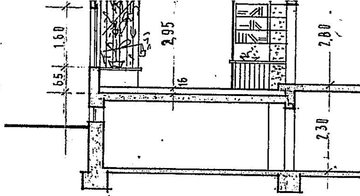
SCHNITT A-A
