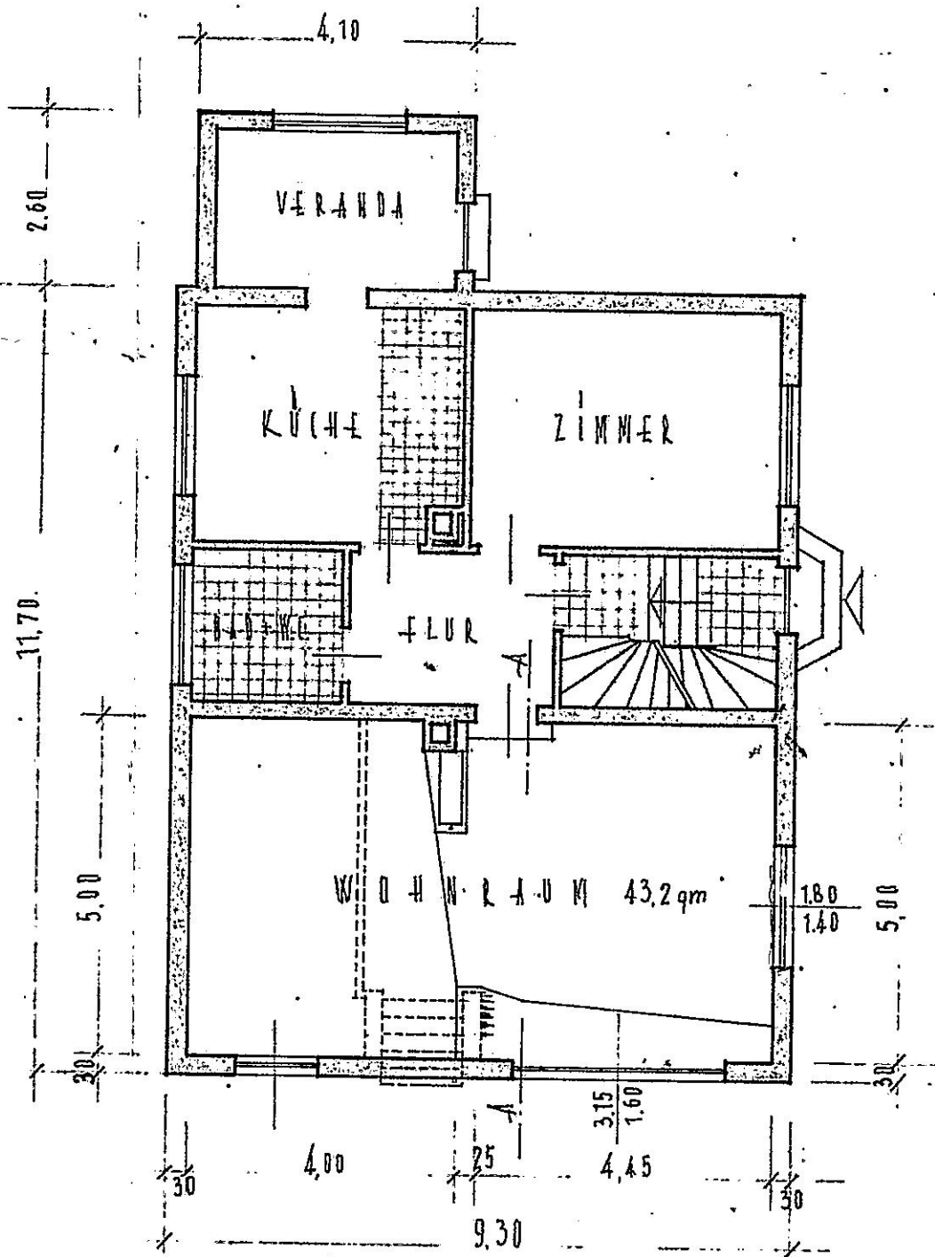
ERDGESCHOSS
