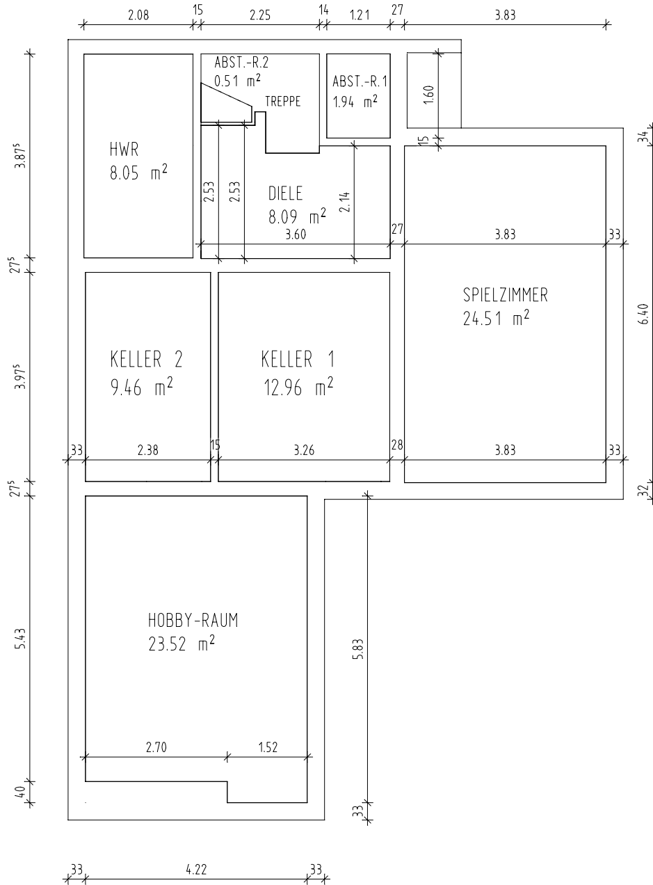
ÜBERSICHT: GRUNDRISS KELLERGESCHOSS
