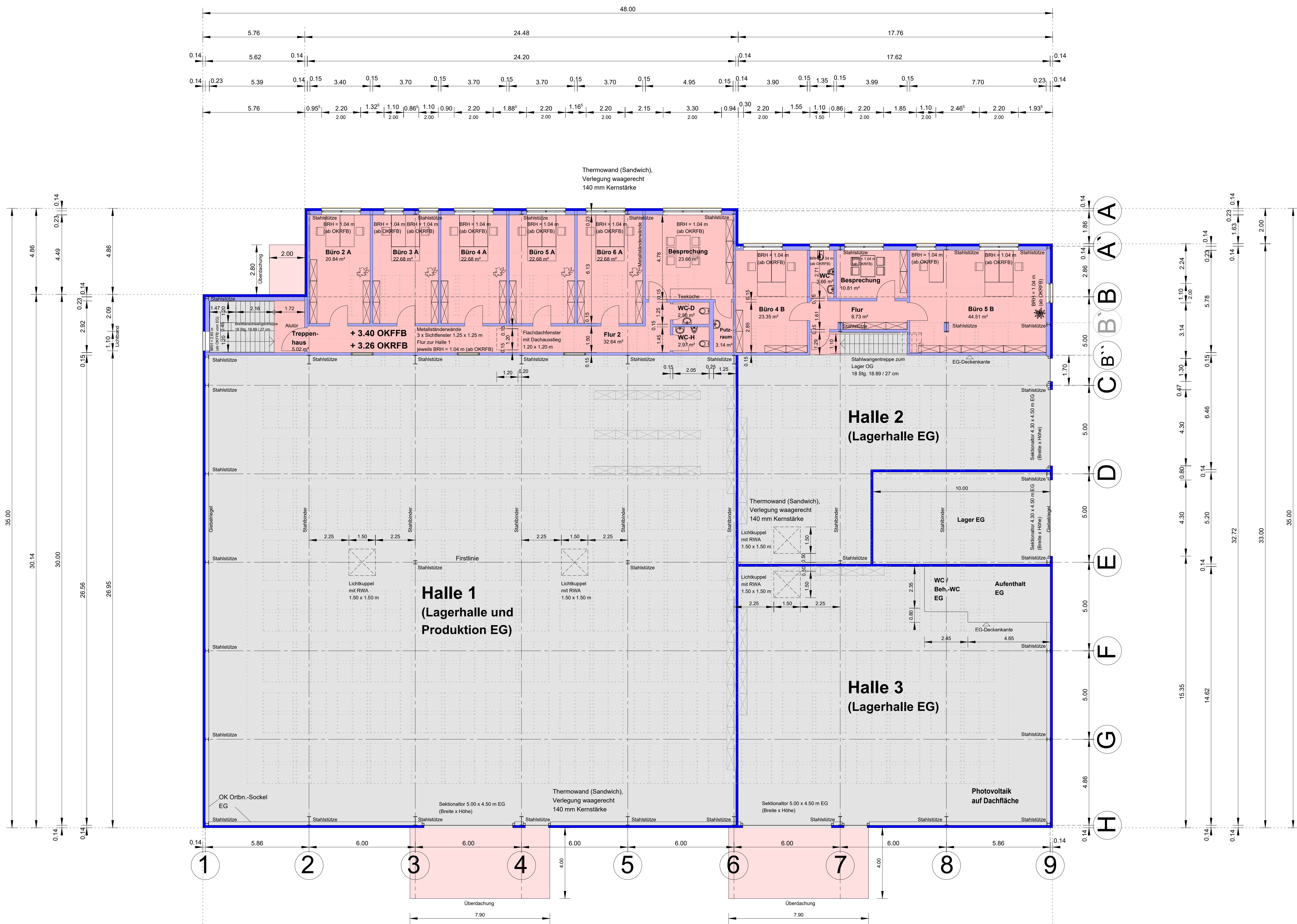
Grundriss Obergeschoss
