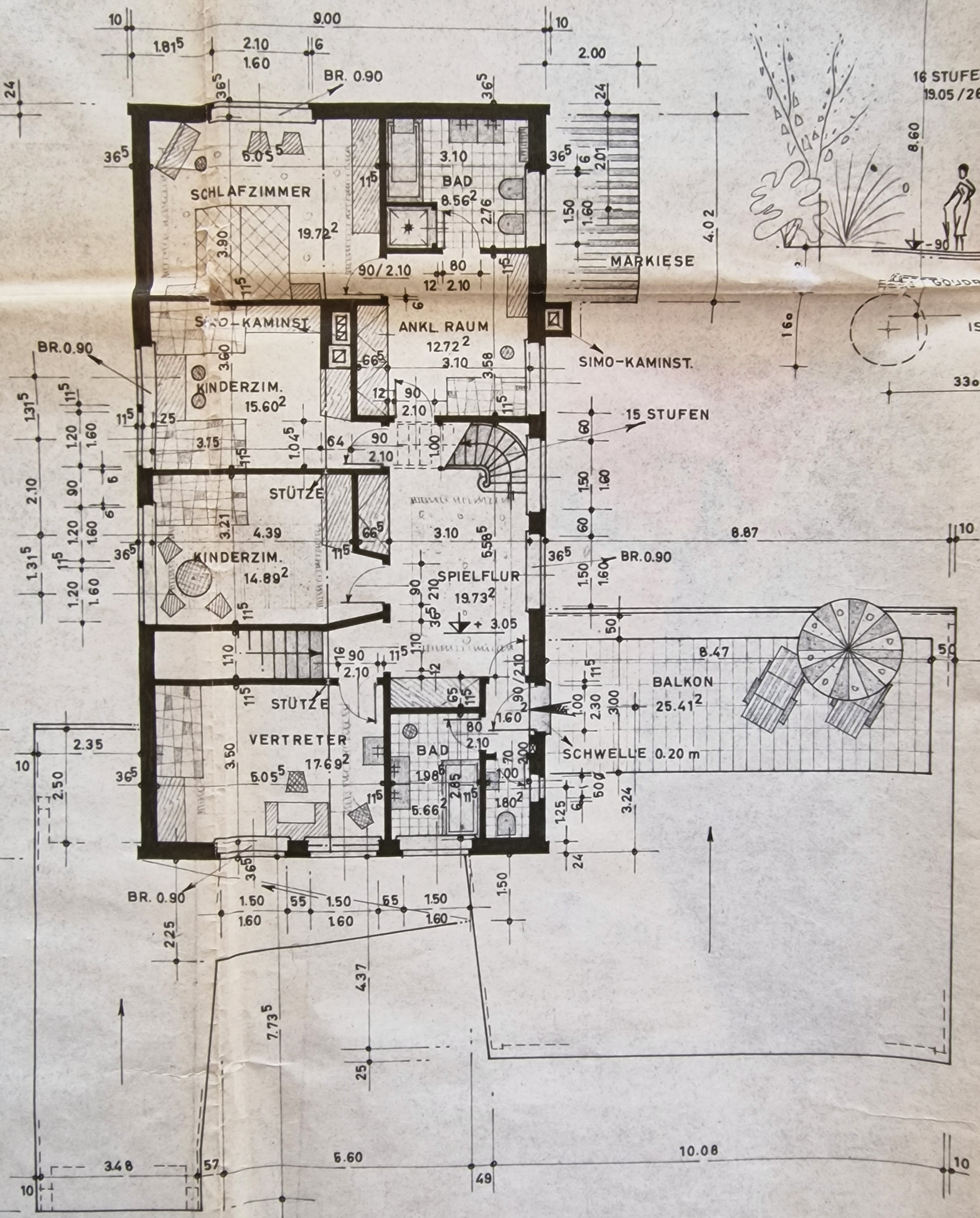
DAS I. OBERGESCHOSS HÖHE 2.95 m
