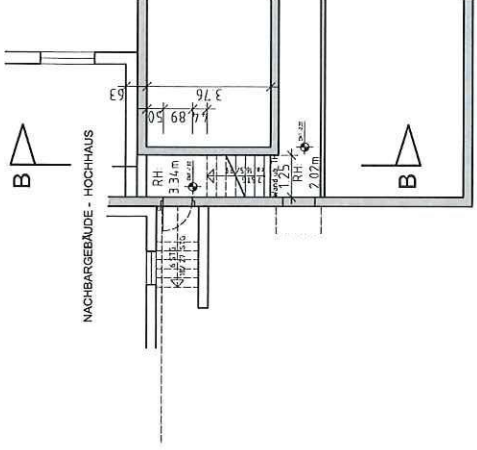
TEILGRUNDRISS KG ZUGANG KELLER/ ANSCHLUSS AN NACHBARGEBAUDE
