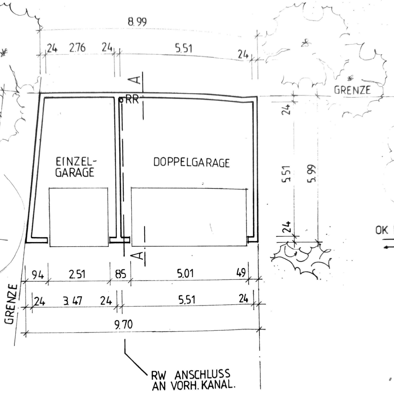
GRUNDRISS
