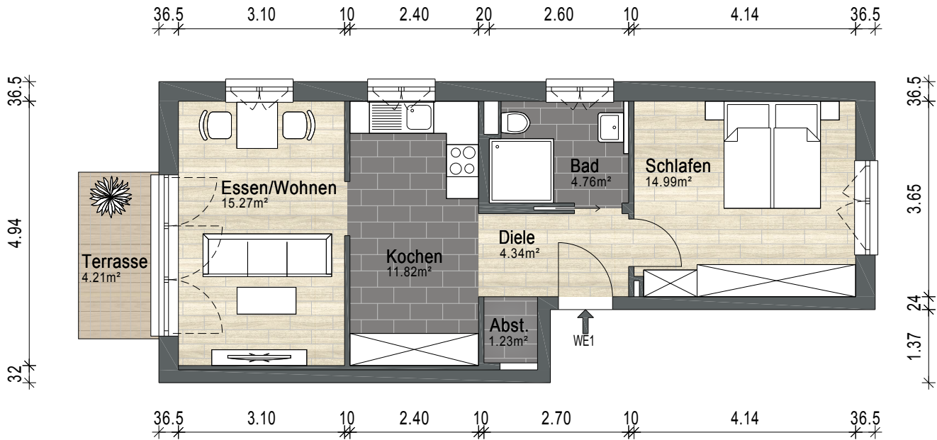
Erdgeschoss
