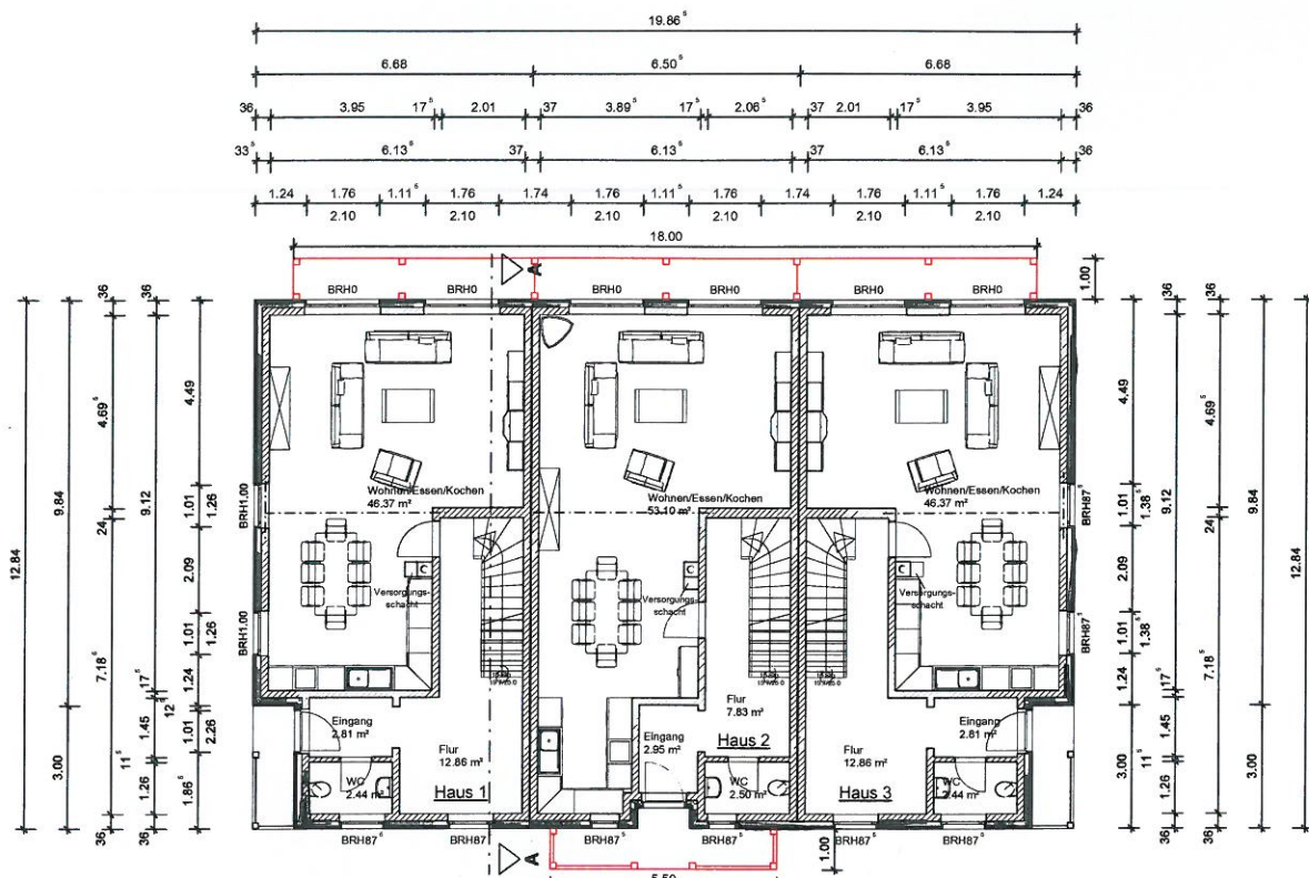
Erdgeschoss
