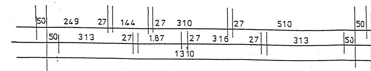
Grundriß Kellergeschoß
