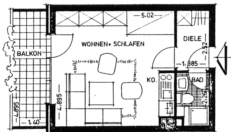
GRUNDRISS M. 1:100 \nabla
