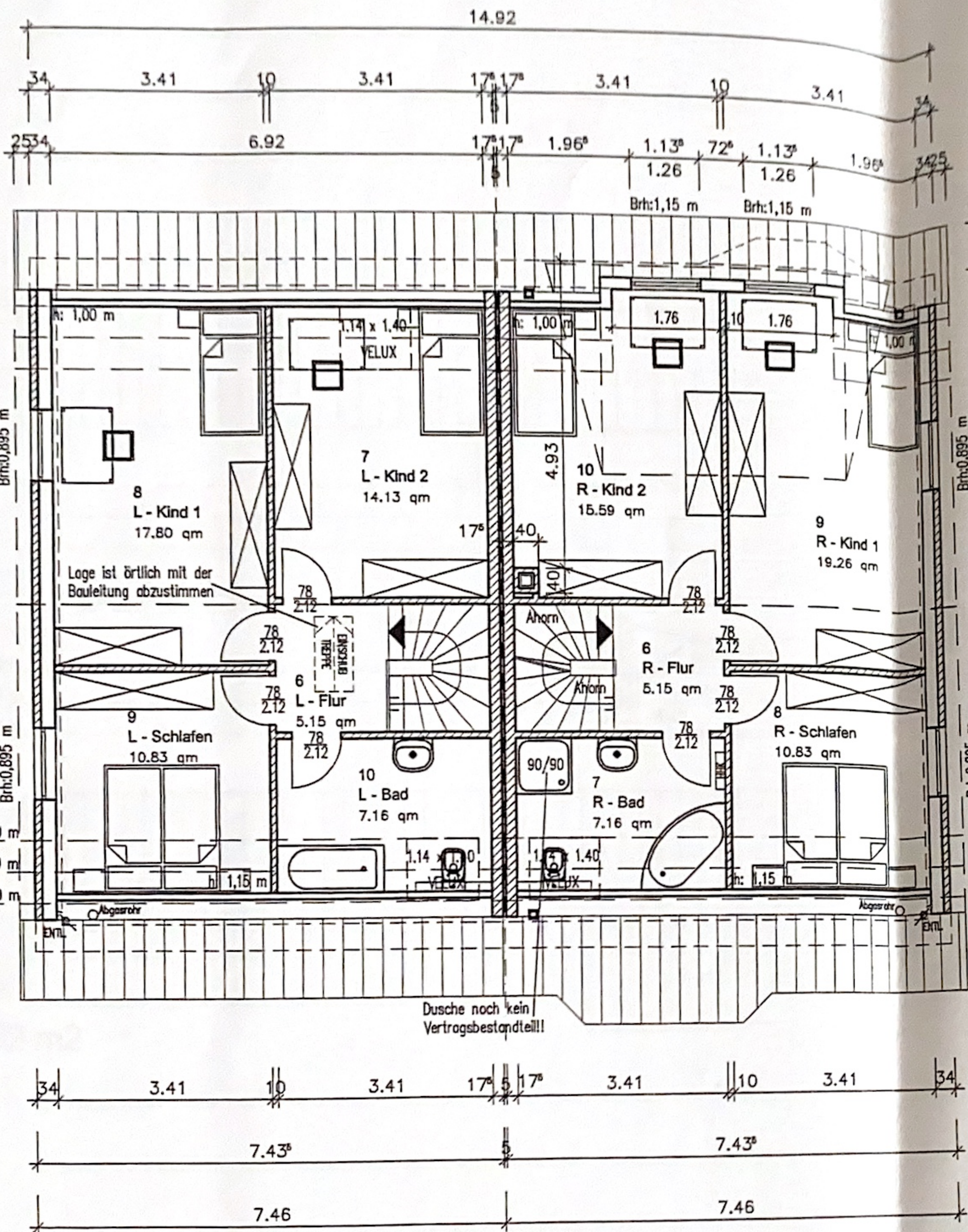
DACHGESCHOSS M 1:100
