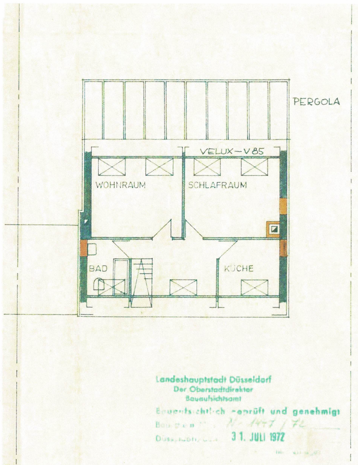
GRUNDRISS DACHGESCHOSS
