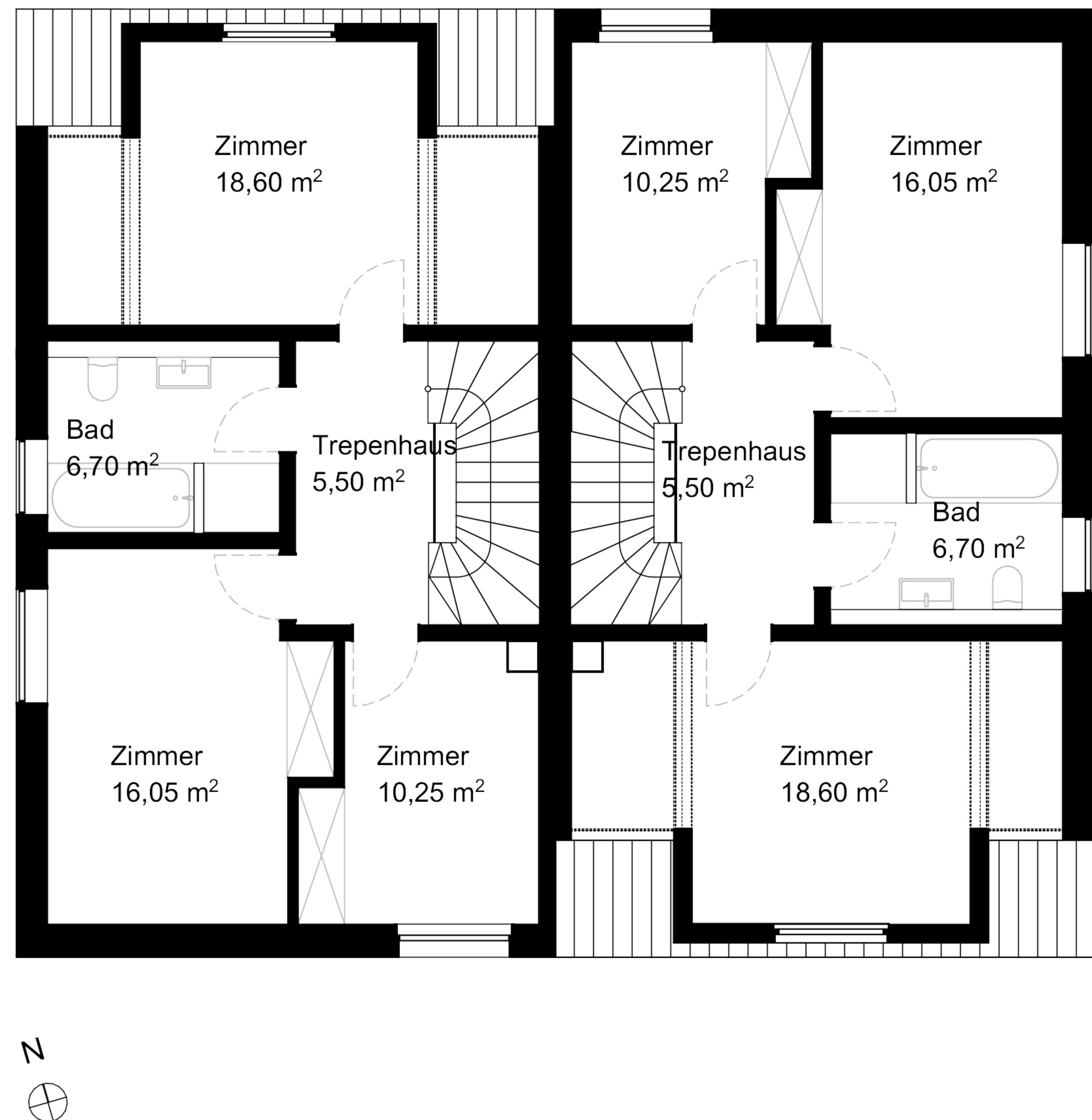
Grundriss OG
