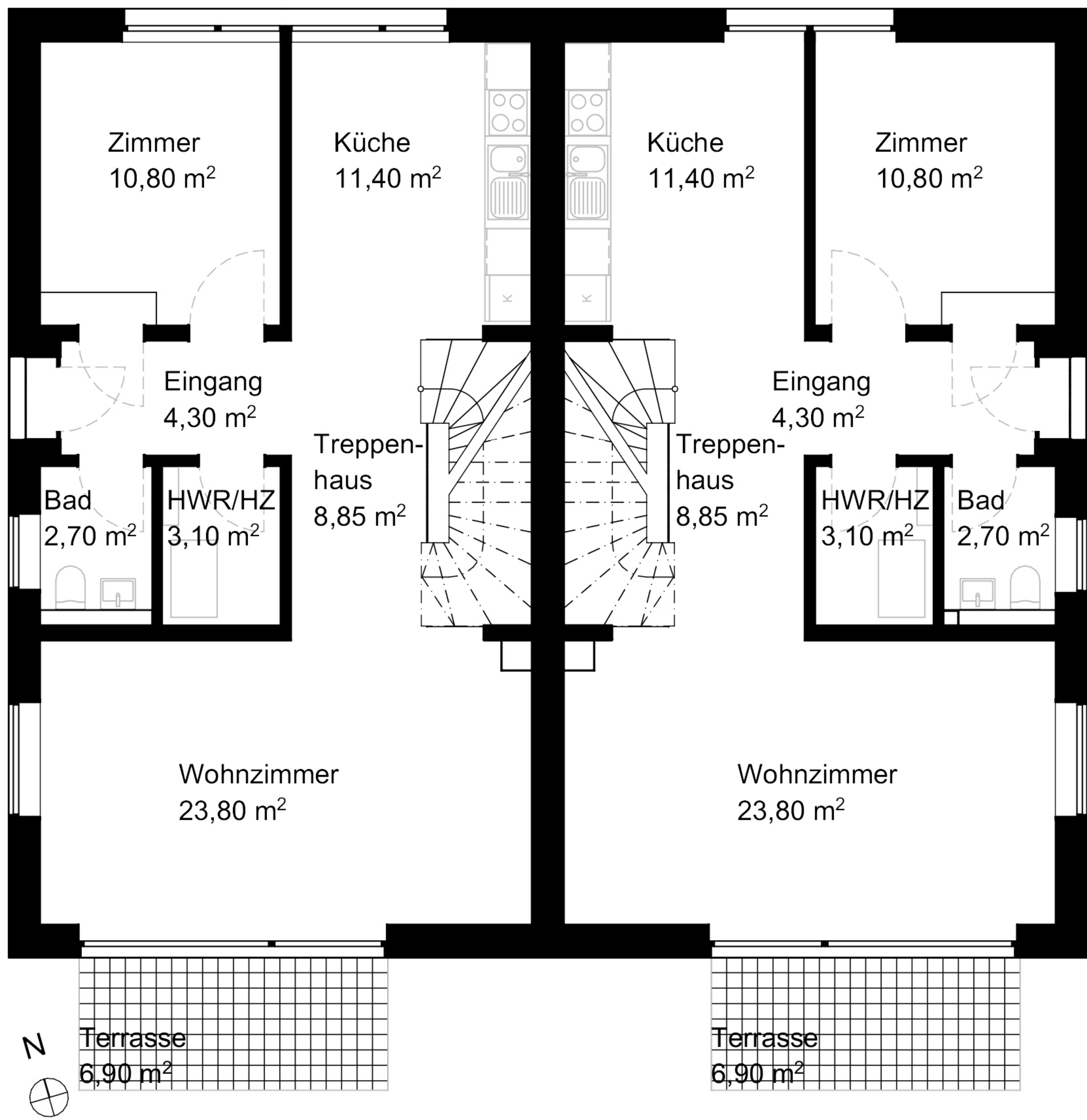
Grundriss EG
