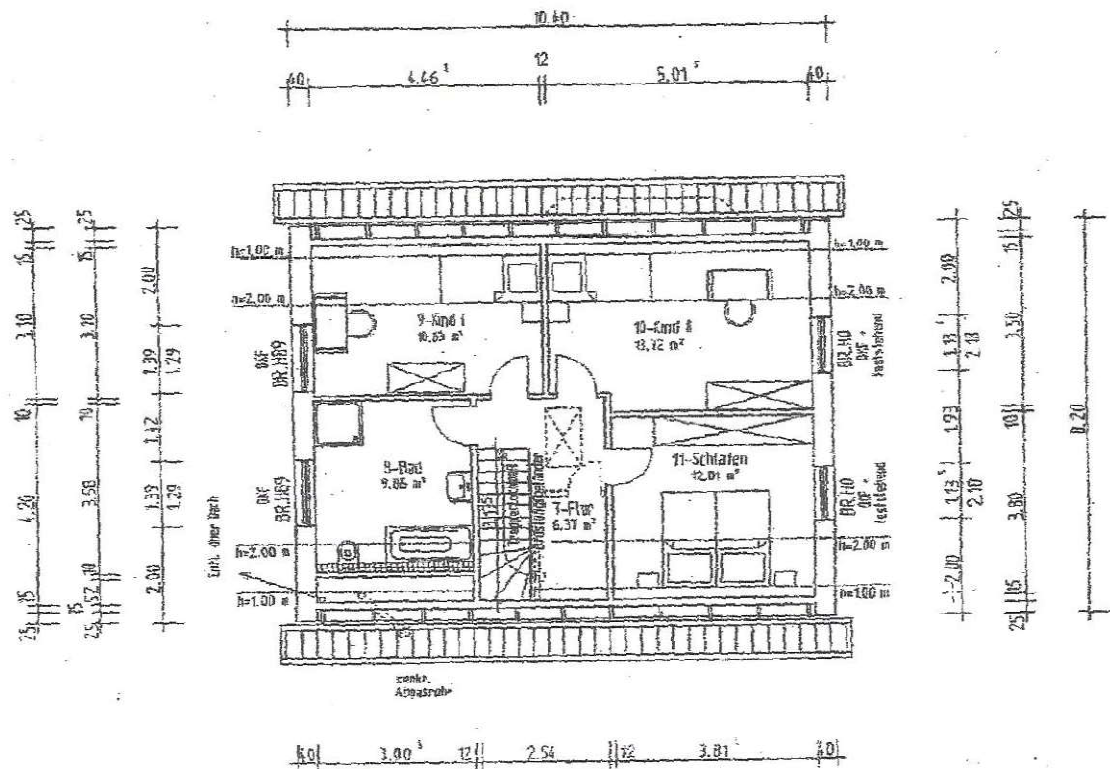
Grundriss Dachgeschoss:
