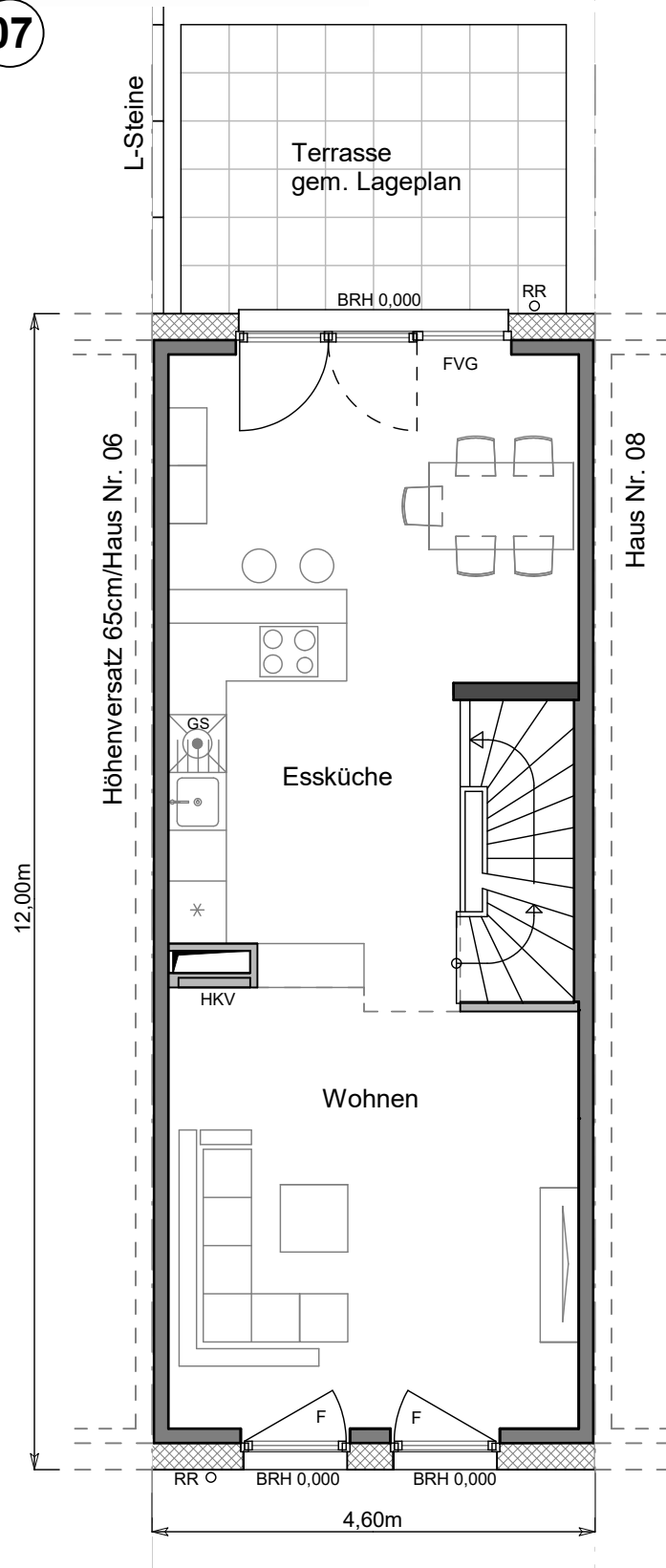
GARTENGESCHOSS M 1:75/DIN A4 alternative Kucheneinteilung
