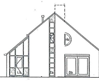
achtergevel
