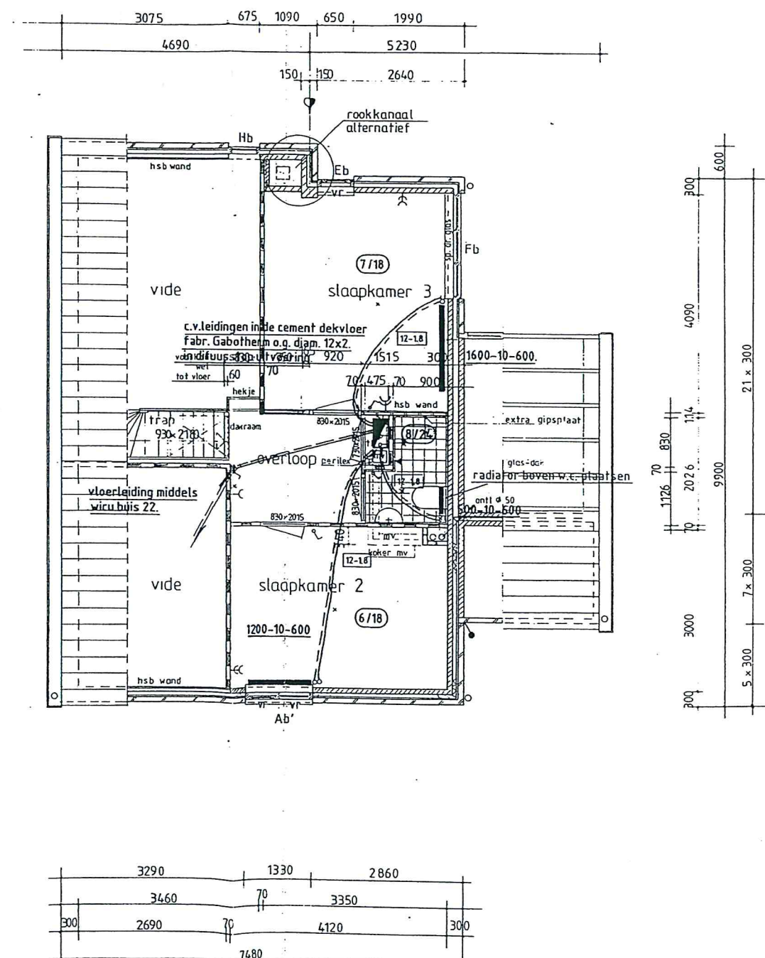
verdieping
