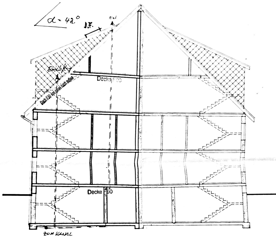
SCHNITT A-A
