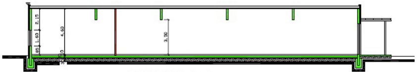
SCHNITT A-A
