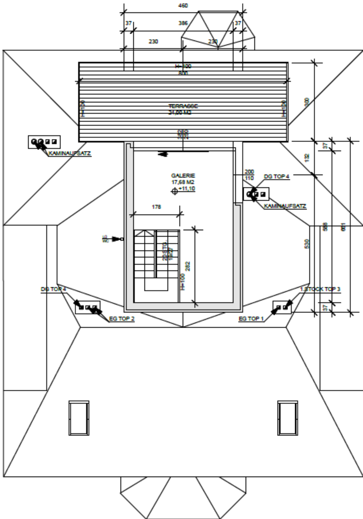
GALERIE, M=1:100
