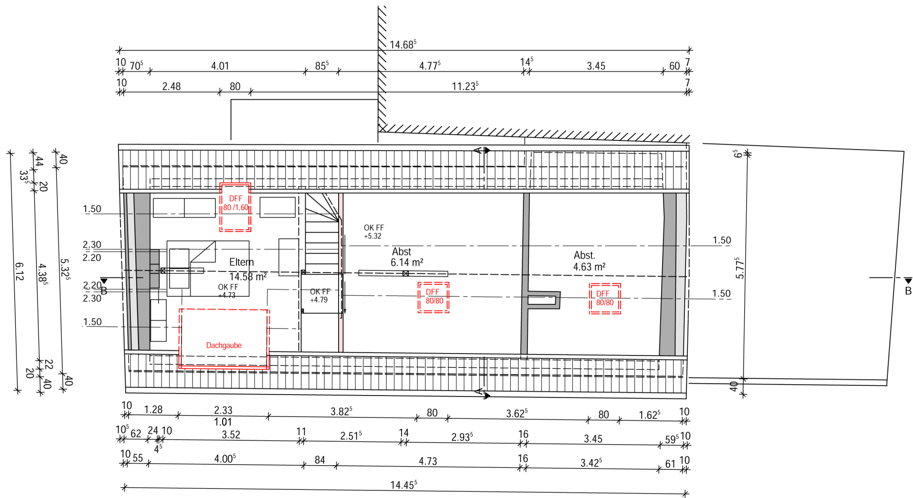
Dachgeschoss Neuplanung
