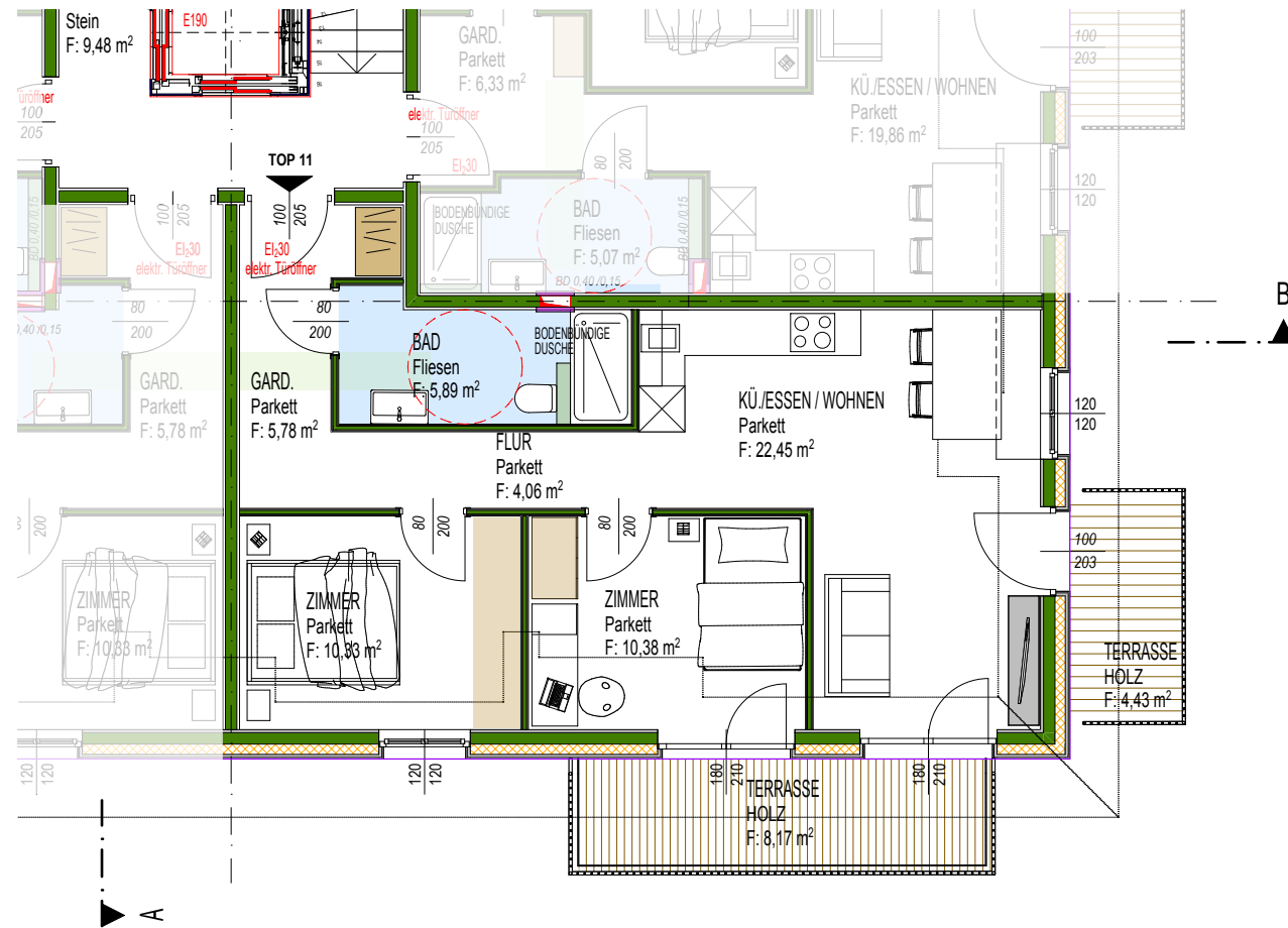
2.OBERGESCHOSS 1:100
