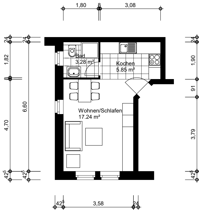
Grundriss
