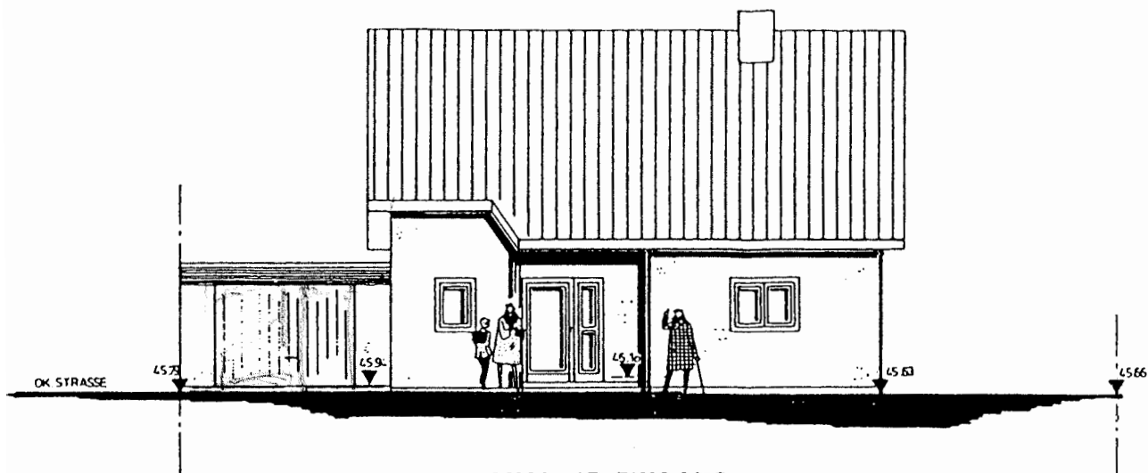
ANSICHT EINGANG
