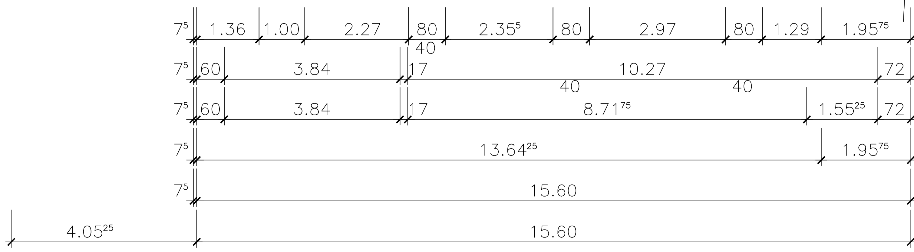
KELLERGESCHOSS BESTAND / NEUPLANUNG M 1 : 50
