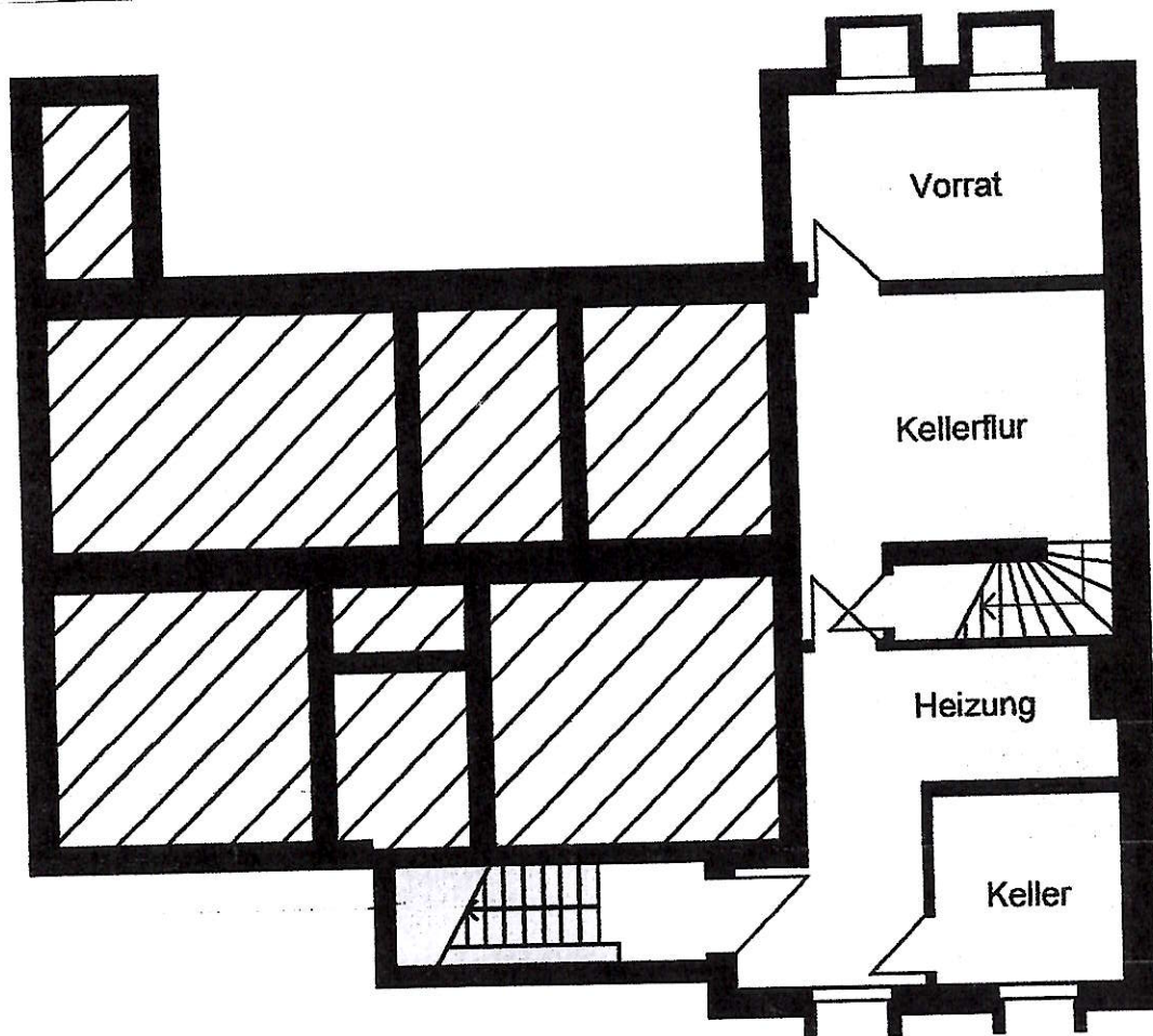
Grundriss Keller
