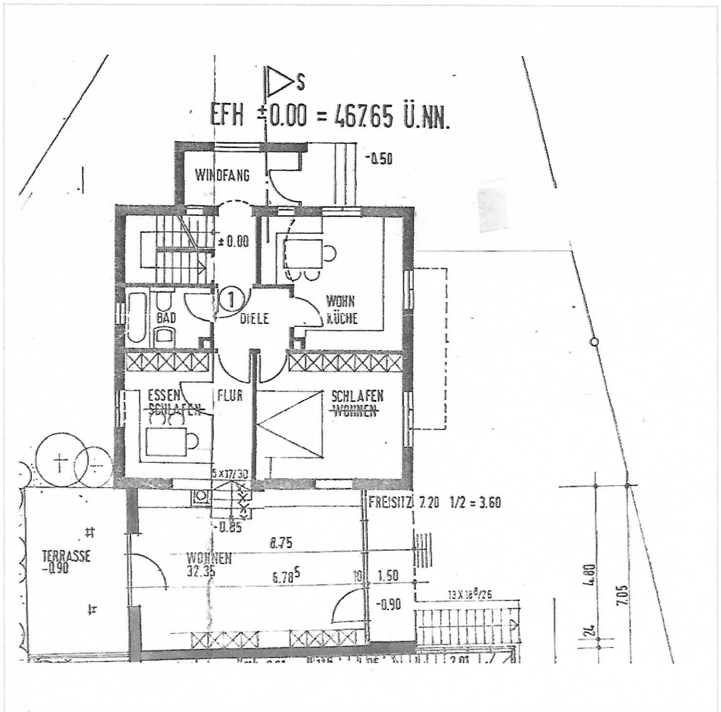
Grundriss EG
