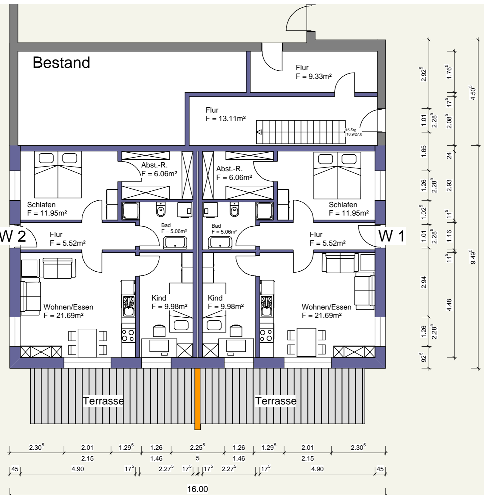
Grundriß Erdgeschoss
