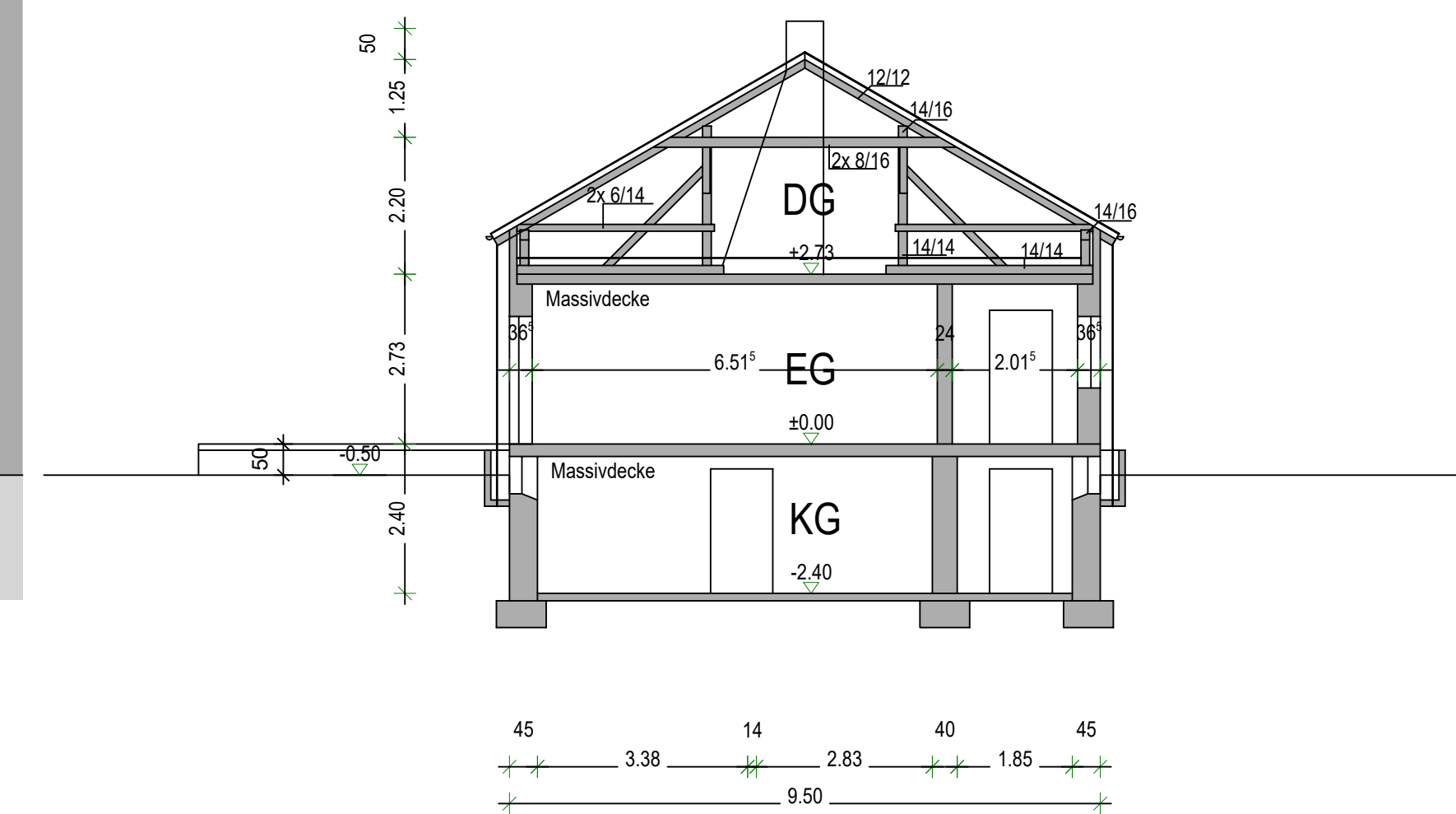
Schnitt B-B Zwischenbau
