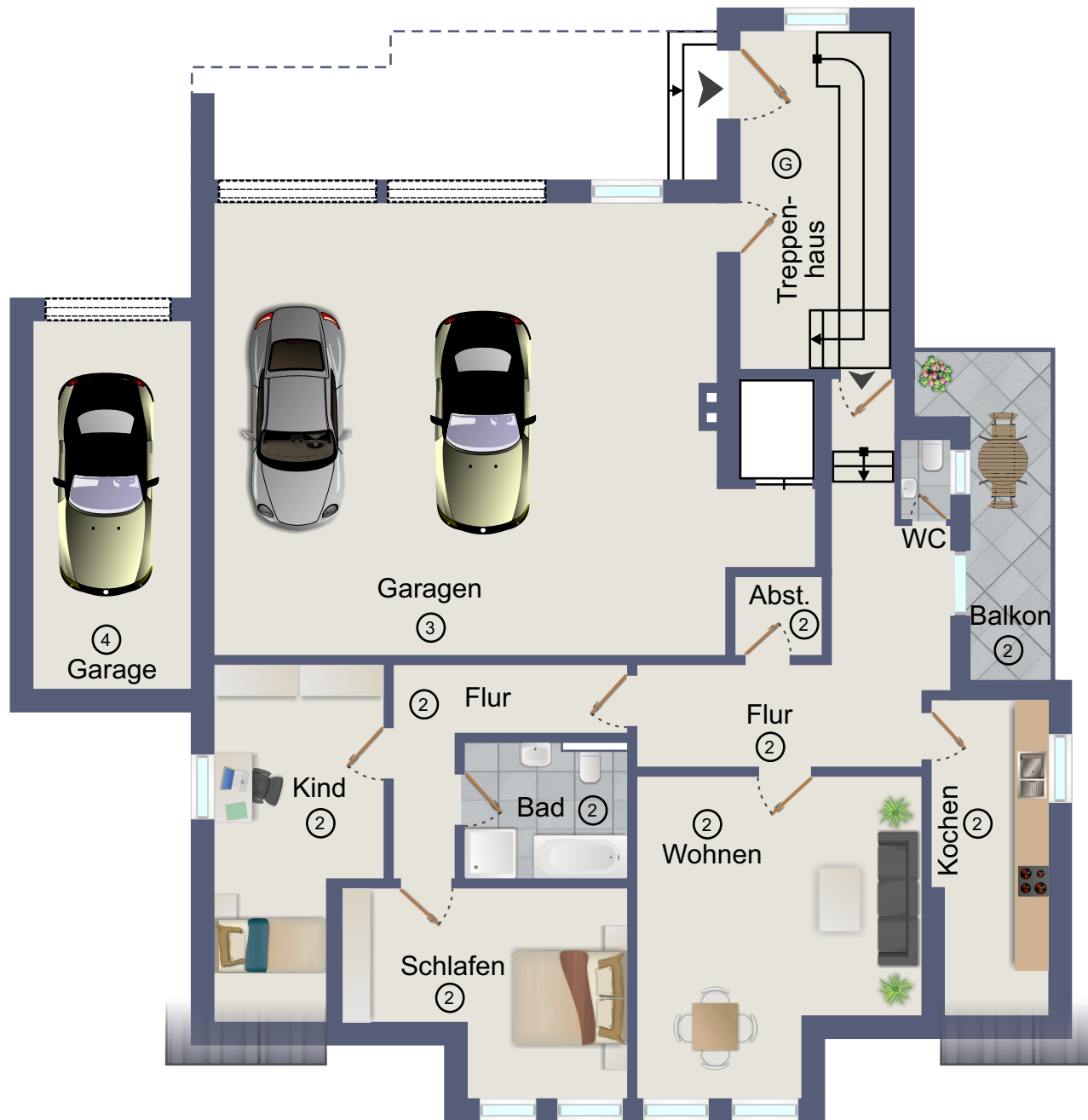
Erdgeschoss
