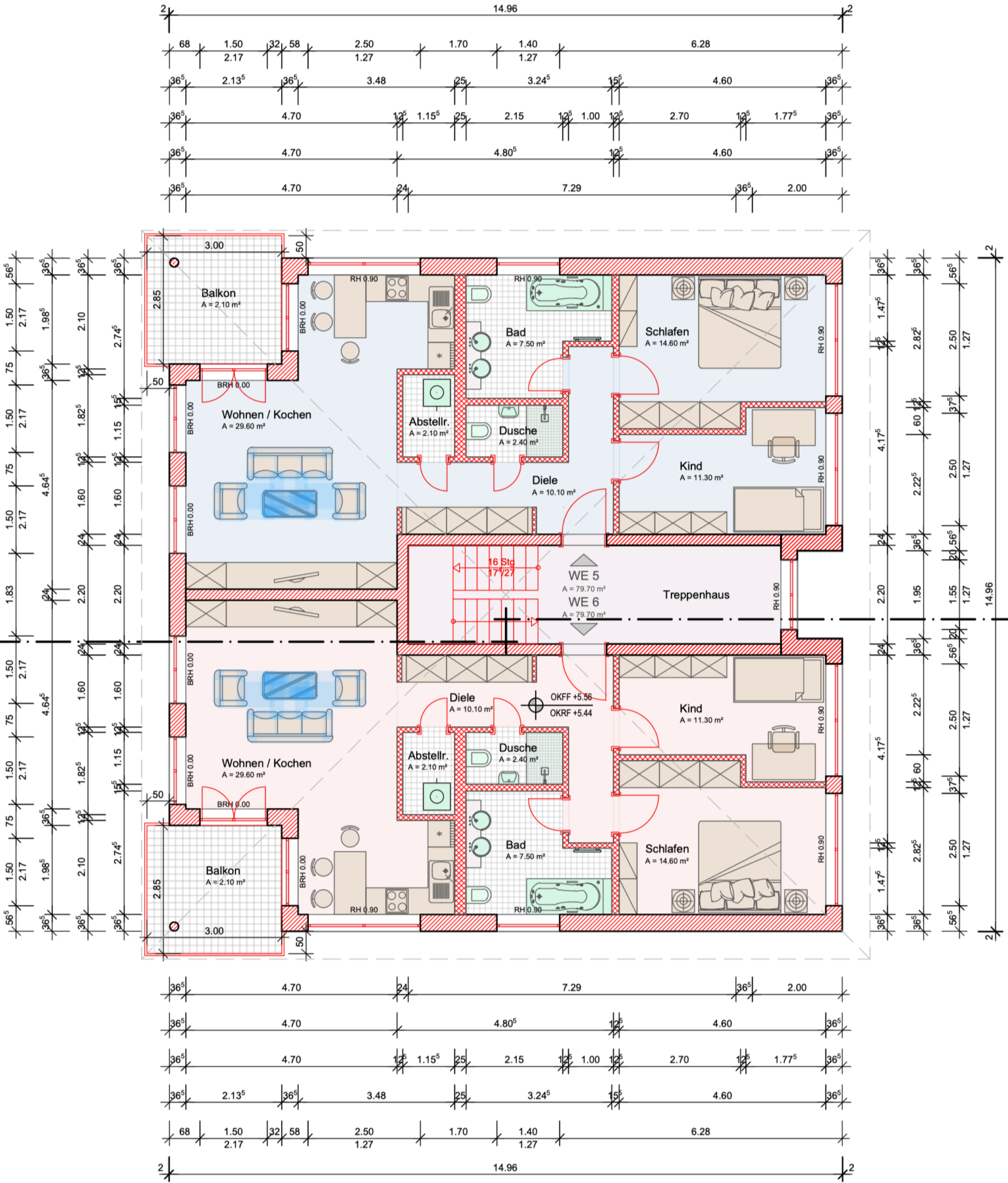
Grundriss Dachgeschoss
