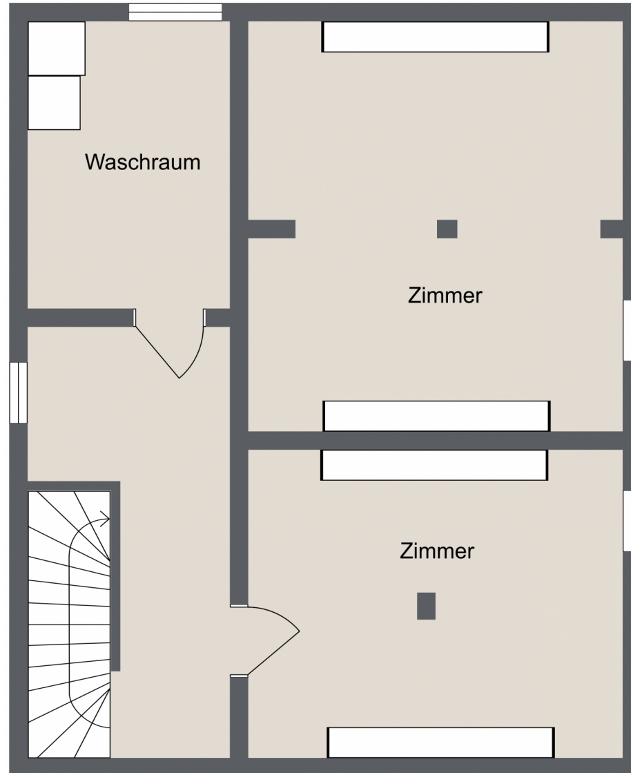
Kellergeschoss
