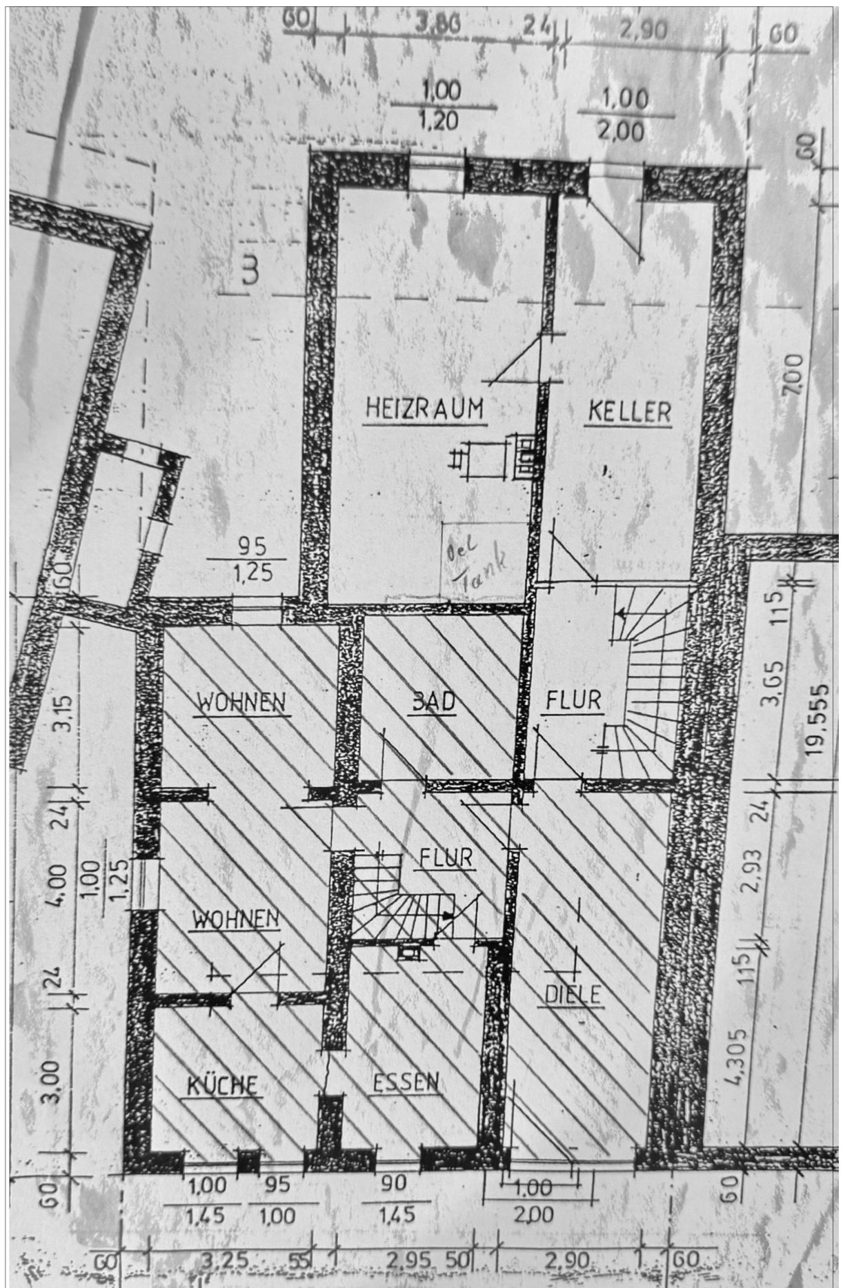
GRUNDRISS ERDGESCHOSS.
