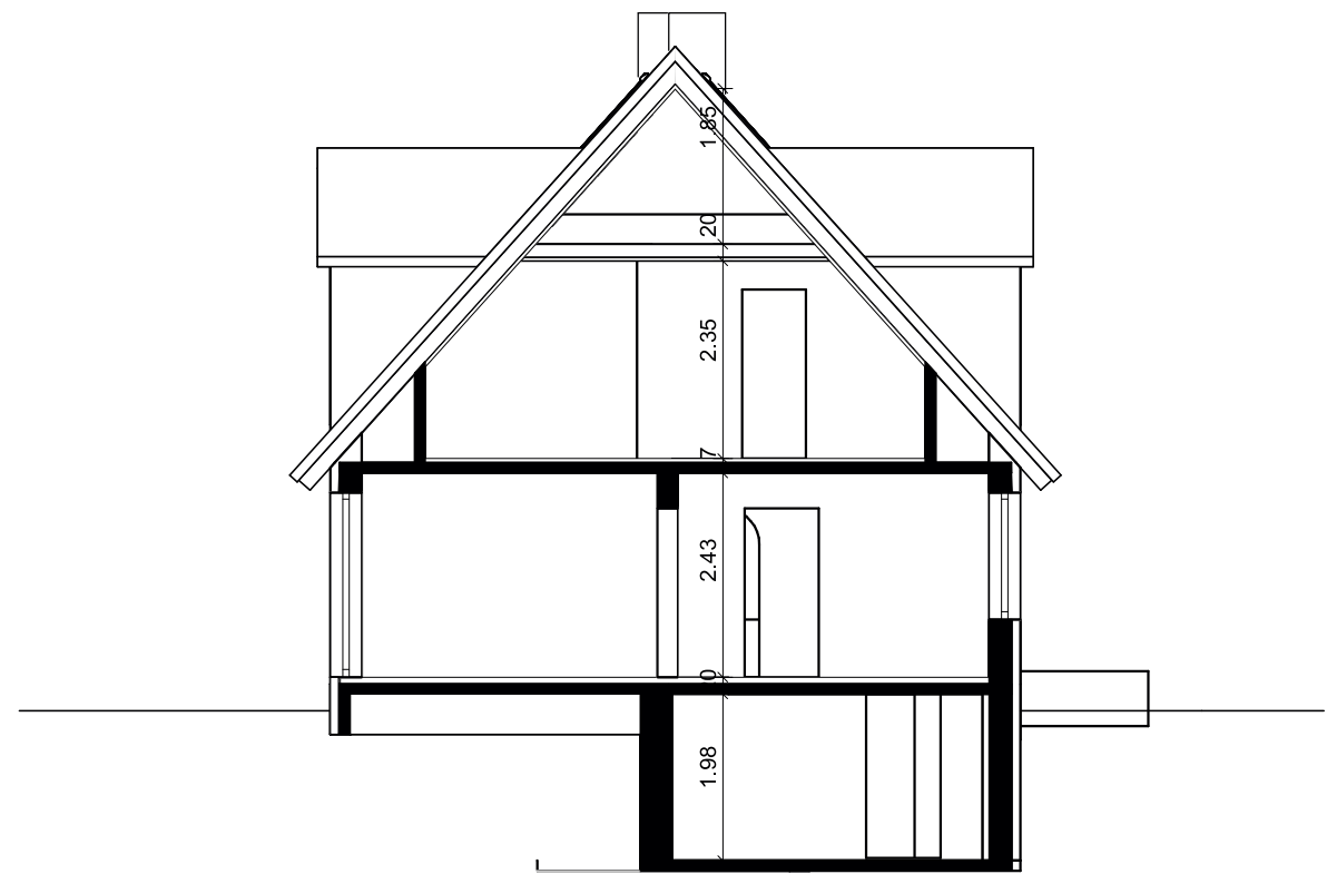
SCHNITT A-A
