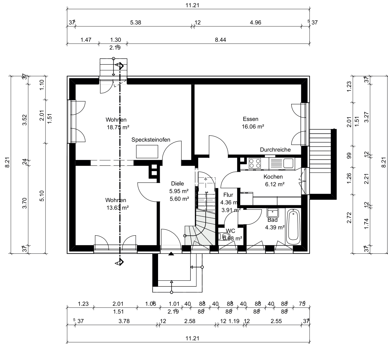
ERDGESCHOSS
