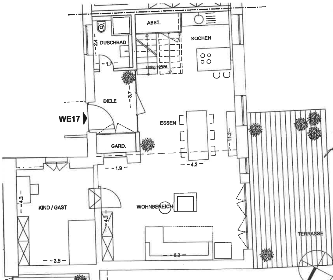
ERDGESCHOSS
