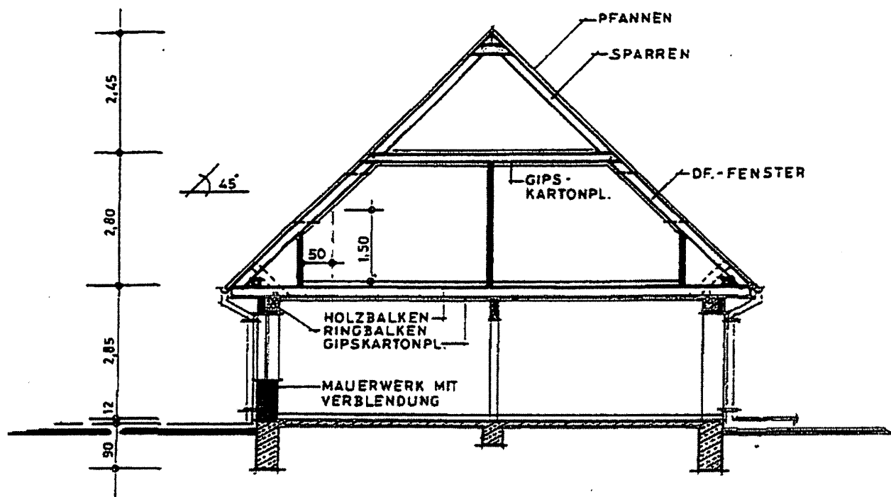
SCHNITT A-B
