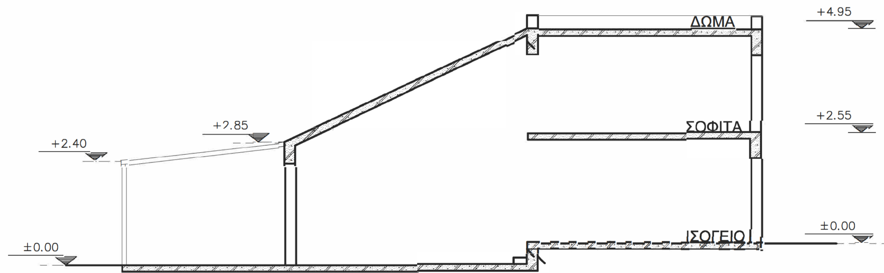
ΣΧΗΜΑΤΙΚΗ ΤΟΜΗ ΚΤΙΡΙΩΝ "Β" & "Γ"
