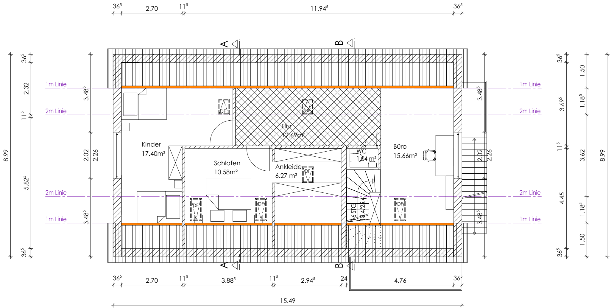
Grundriss-Dachgeschoss
