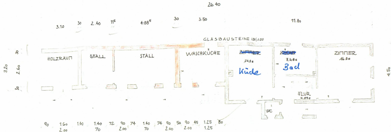
ERDGESCHOSSGRUNDRISS , NEU
