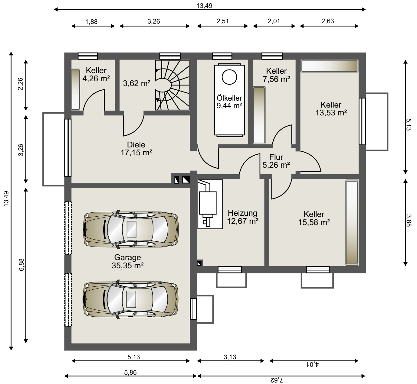
Kellergeschoss
