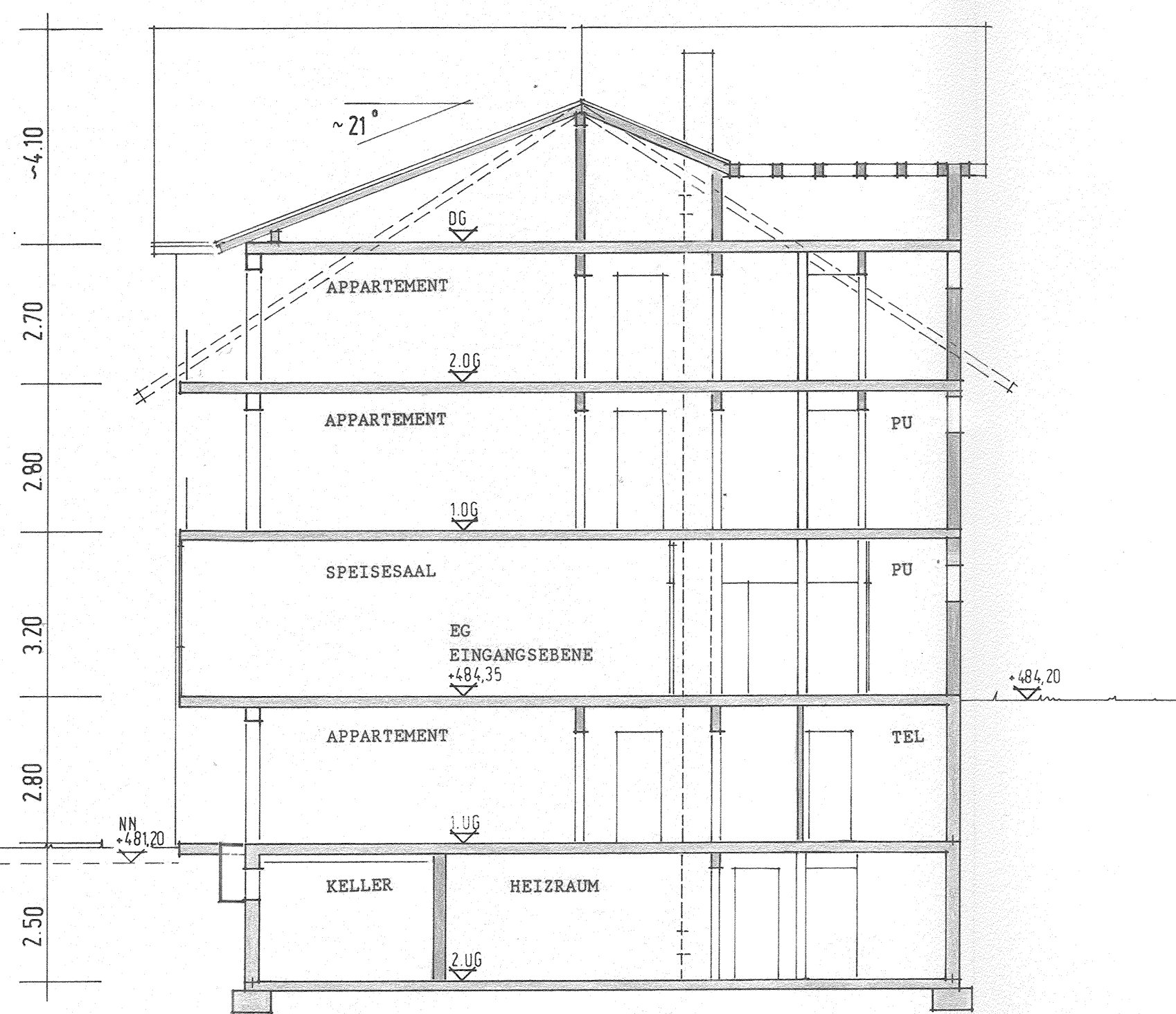
SCHNITT A-A
