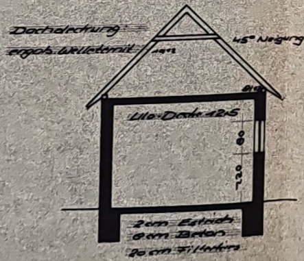
Schnitt
