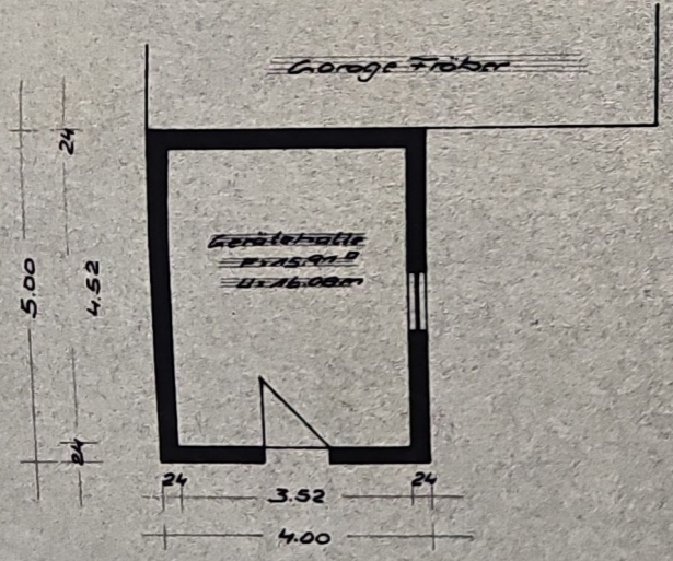
Grundriss
