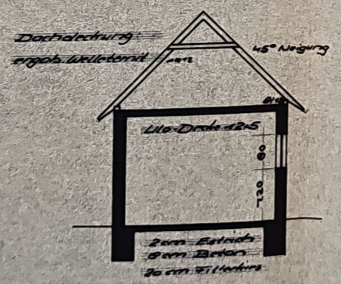
Schnitt
