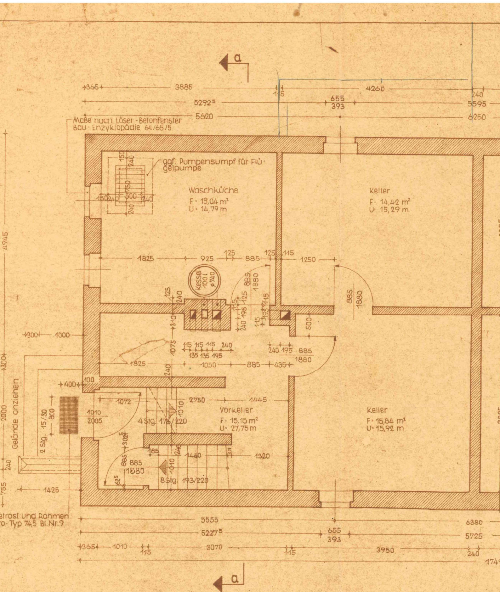
KELLERGECHOSS-GRUNDRISS
