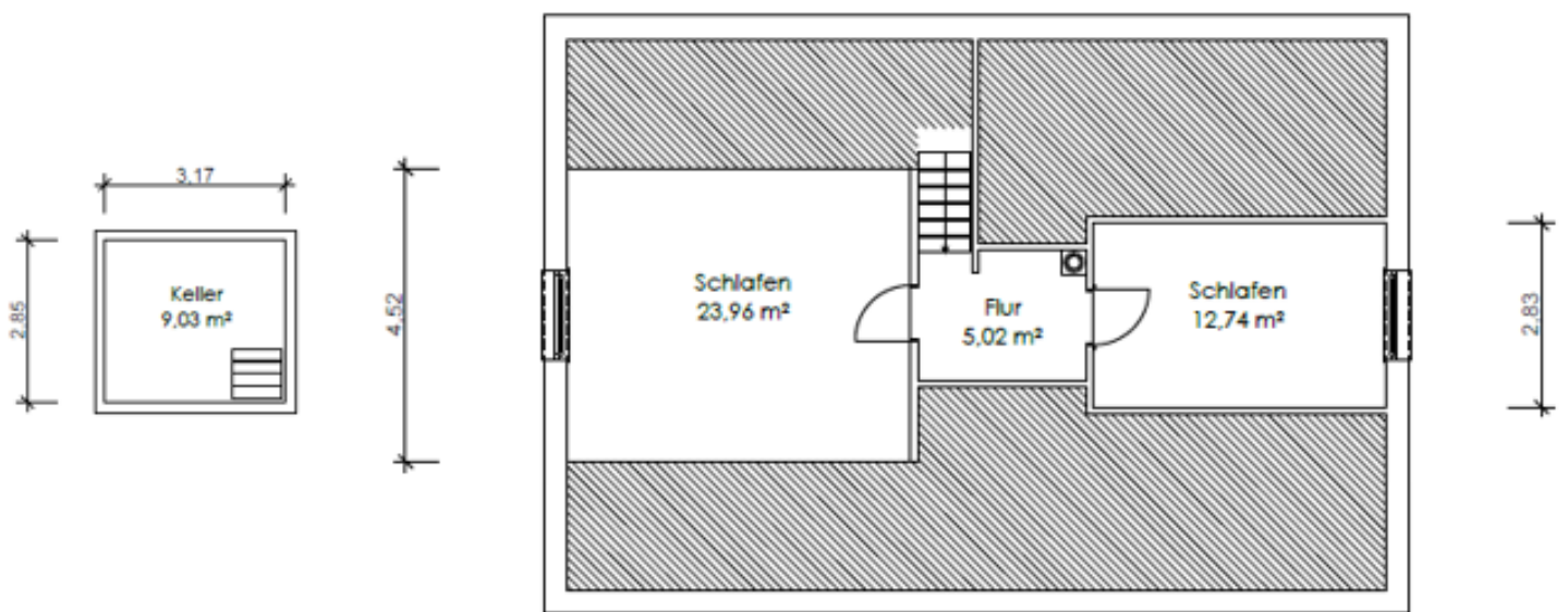
Grundriss OG
