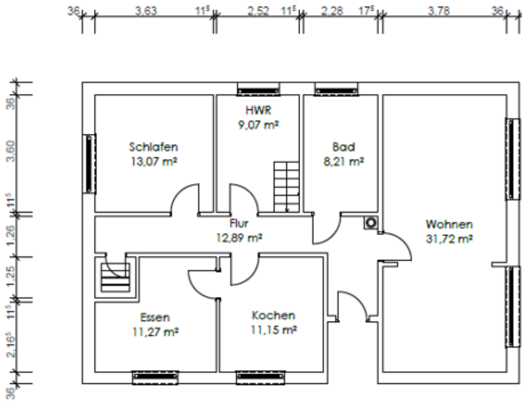
Grundriss EG
